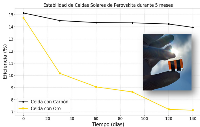
Figura 5. Monitoreo de la estabilidad para celdas solares de perovskita, con dos contactos diferentes: Carbón (puntos negros) y Oro (puntos amarillos), durante 5 meses (elaboración propia)
