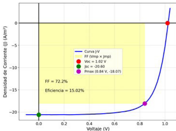
Figura 4. Curva Densidad de corriente contra Voltaje (J-V) para una celda solar de perovskita con contactos de carbón, medida bajo una intensidad de iluminación igual a 1 Sol. Los círculos: verde, morado y rojo señalan la densidad de corriente, potencia máxima y voltaje de circuito abierto
