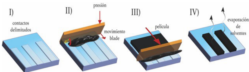
Figura 3. Ilustración de la técnica de doctor blade (elaboración propia)
