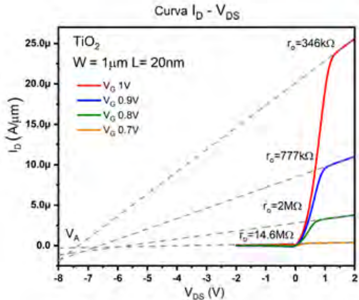
Figura 14 Curvas de corriente de salida I_{DS} - V_{DS} para varios voltajes V_G , obteniendo la resistencia de salida en saturación r_o y voltaje Early V_A para \text{TiO}_2 .
