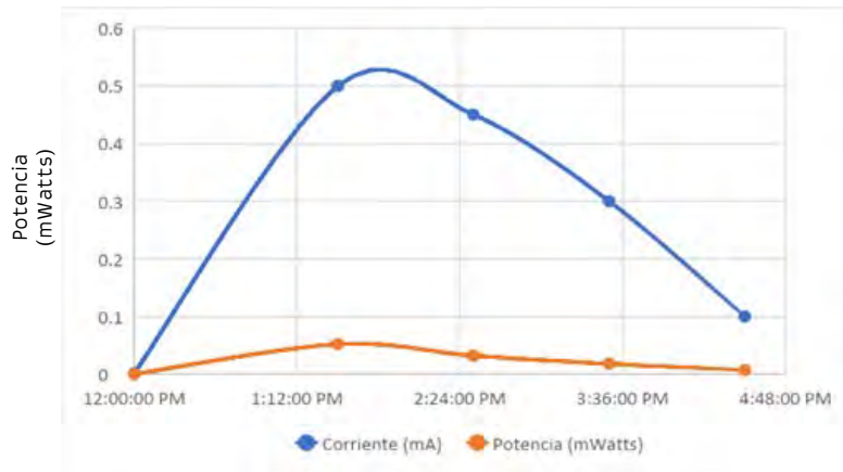
Figura 9. Gráfica de potencia contra corriente generada por la celda.
