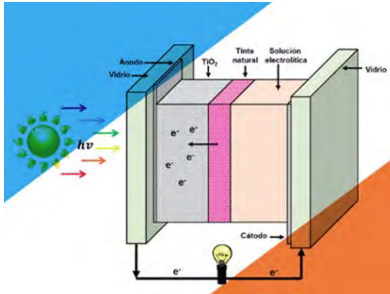
Figura 1. Partes de una celda solar sensibilizada por colorante (Pezzotti-Escobar G, 2015) https://revista.cidet.org.co/revistas/revista-12/celdas-solares-dssc-tecnologia-prometedora-para-la-produccion-de-electricidad-a-bajo-costo/
