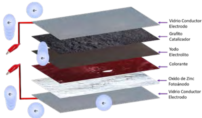
Figura 3. Proceso de elaboración de la celda solar sensibilizada por tinte.
