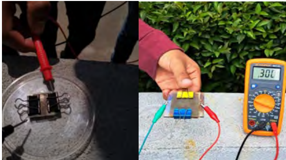
Figura 5. Mediciones de la celda solar a diferentes horas del día. Por Los autores
